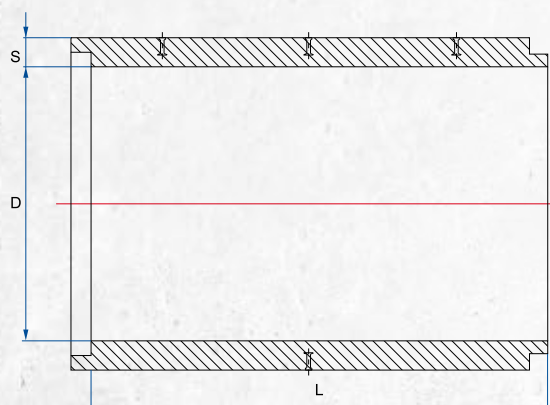
Rura żelbetowa 1500
